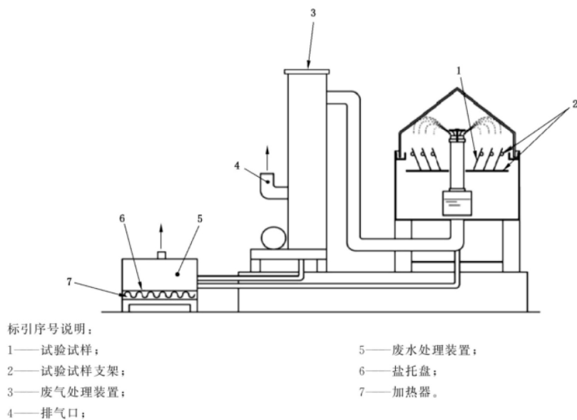
图 C.2 盐雾箱的设计示意图 侧面图
