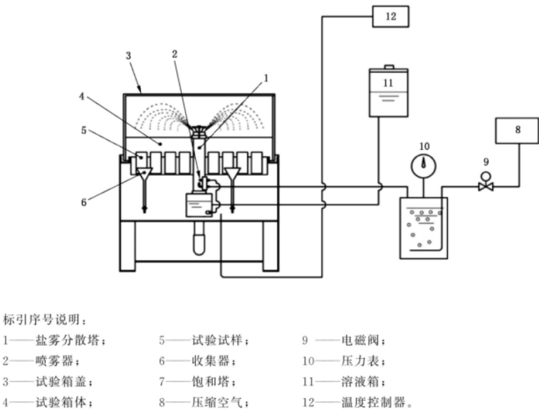
图 C.1 盐雾箱的设计示意图(正面图)
